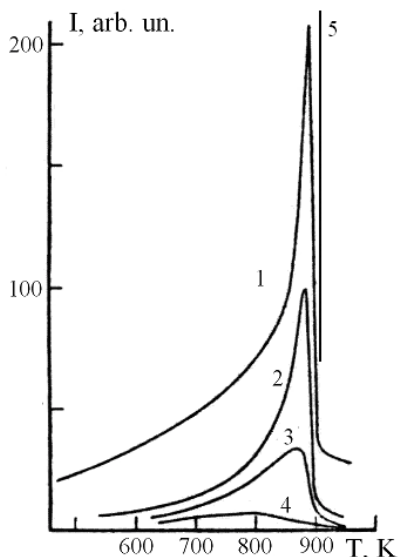
Рис. 3. Изочастотные температурные зависимости рассеяния света в кристаллах танталата лития при геометрии рассеяния X(ZZ)Y на мягкой моде вблизи точки фазового перехода при фиксированных частотах ( \omega = 2, 4, 16 и 86 \text{ см}^{-1} соответственно). Сплошная линия (5) при T = T_c = 898 \text{ К} соответствует центральному пику рассеянного света
