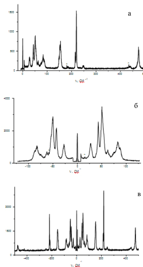
Рис. 2. Вид спектра КР на решеточных и внутримолекулярных модах кристаллической серы; а – стоксов спектр КР; б – низкочастотный участок стоксова и антистоксова КР, соответствующий решеточным модам; в – полный стоксов и антистоксов спектры КР первого порядка
