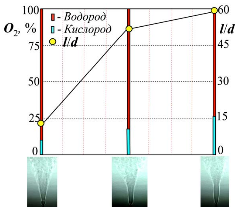
Рис. 9. График изменения размера ( l/d ) и формы (от сферической к цилиндрической) области перетяжки пламени в зависимости от доли кислорода в смеси при скорости истечения круглой микроструи U_0 = 561 м/с и теневые картины процесса горения
