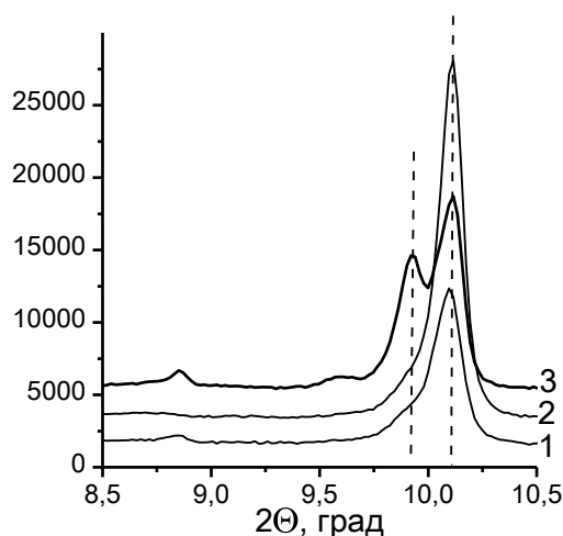
Рис. 3. Дифрактограмма осадков КВЦ с декстраном.
